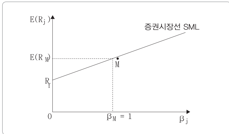
증권시장선 (SML)
